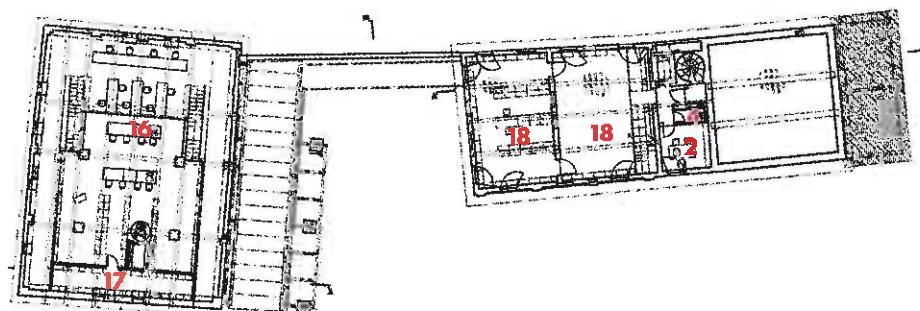
pianta del secondo piano/ second-floor plan
